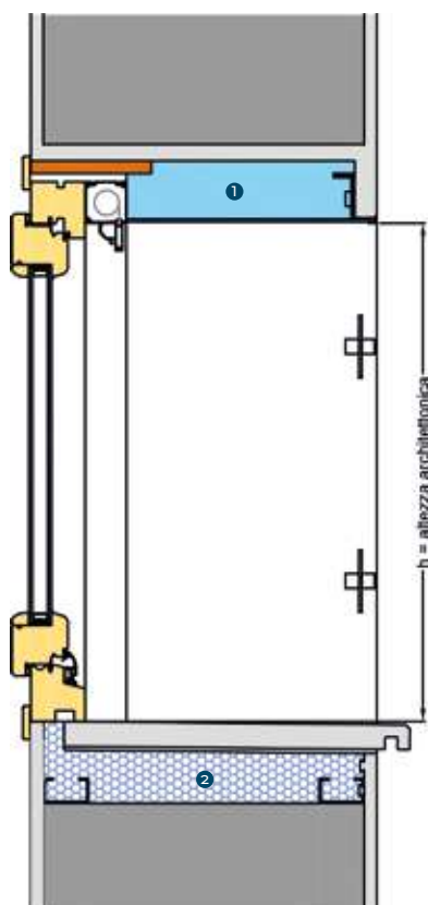
SEZIONE VERTICALE
