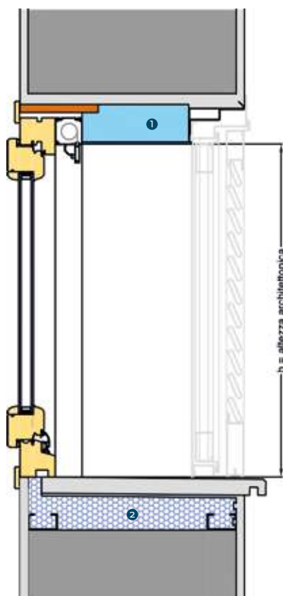
SEZIONE VERTICALE
