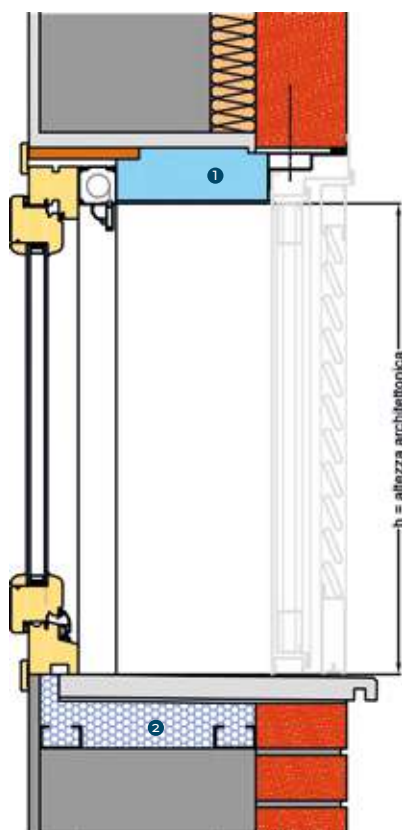
SEZIONE VERTICALE
