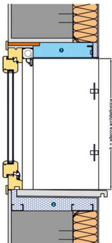
SEZIONE VERTICALE
