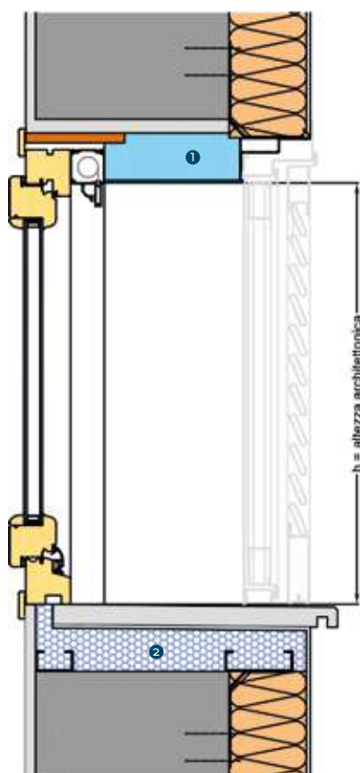
SEZIONE VERTICALE
