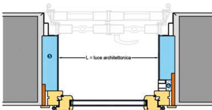
SEZIONE ORIZZONTALE
