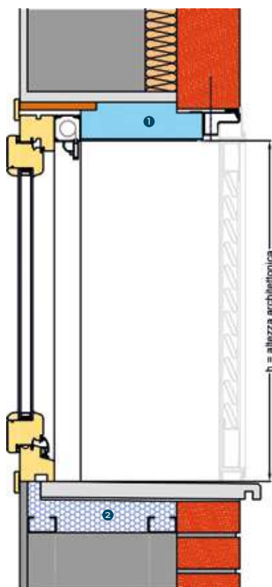
SEZIONE VERTICALE
