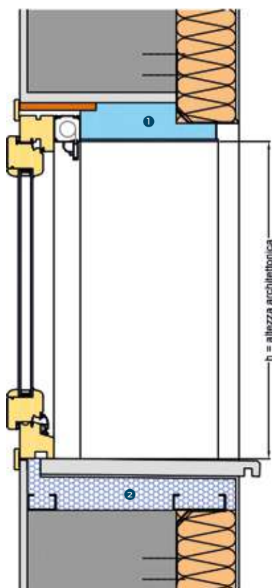
SEZIONE VERTICALE
